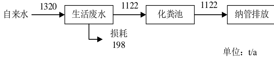
图2-1 水平衡图
