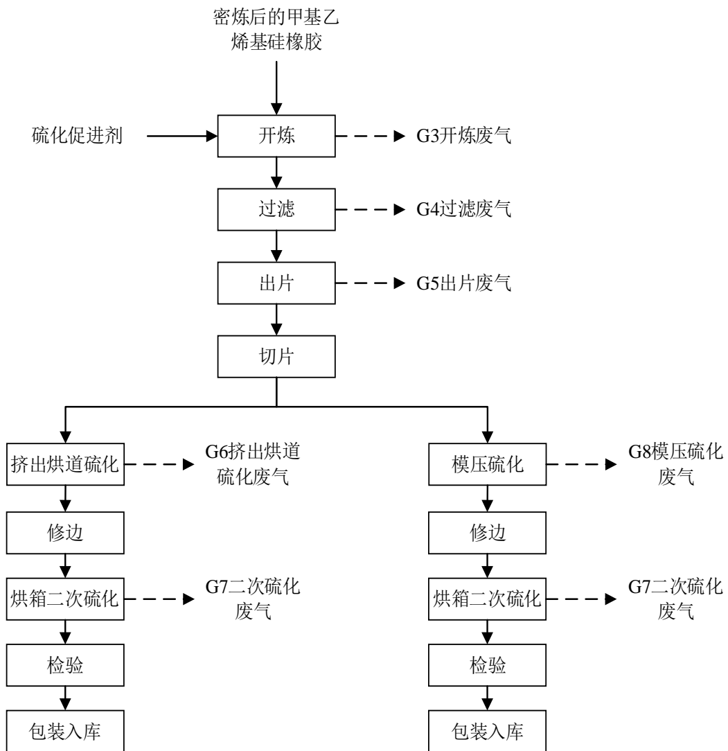
图 2-3 甲基乙烯基硅橡胶产品生产工艺流程及产污图
