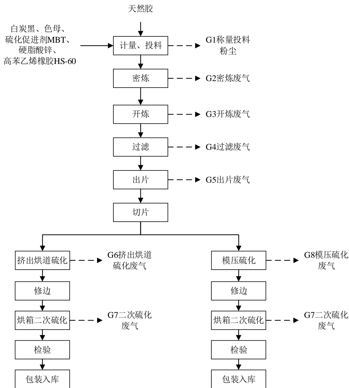
图 2-2 天然胶制品生产工艺流程及产污图
